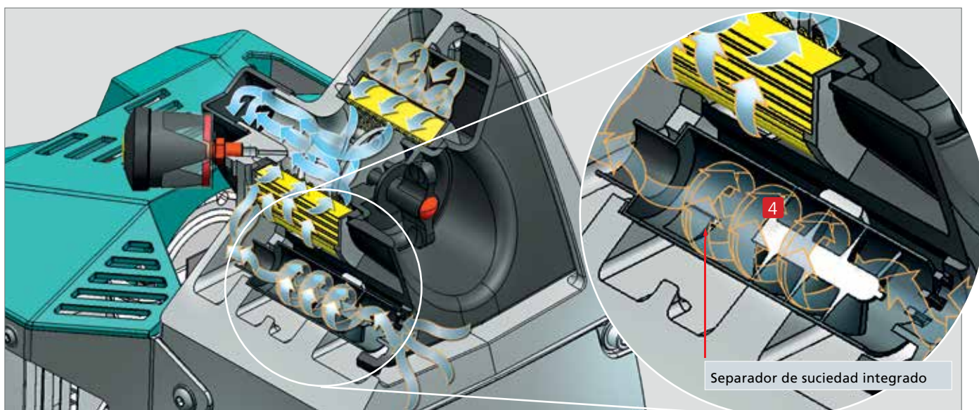
Filtro de aire de gran tamaño y malla fina, fácil de limpiar y opcional con prefiltro ciclón con indicador que aumenta 5 veces más el tiempo de duración del filtro de aire.
